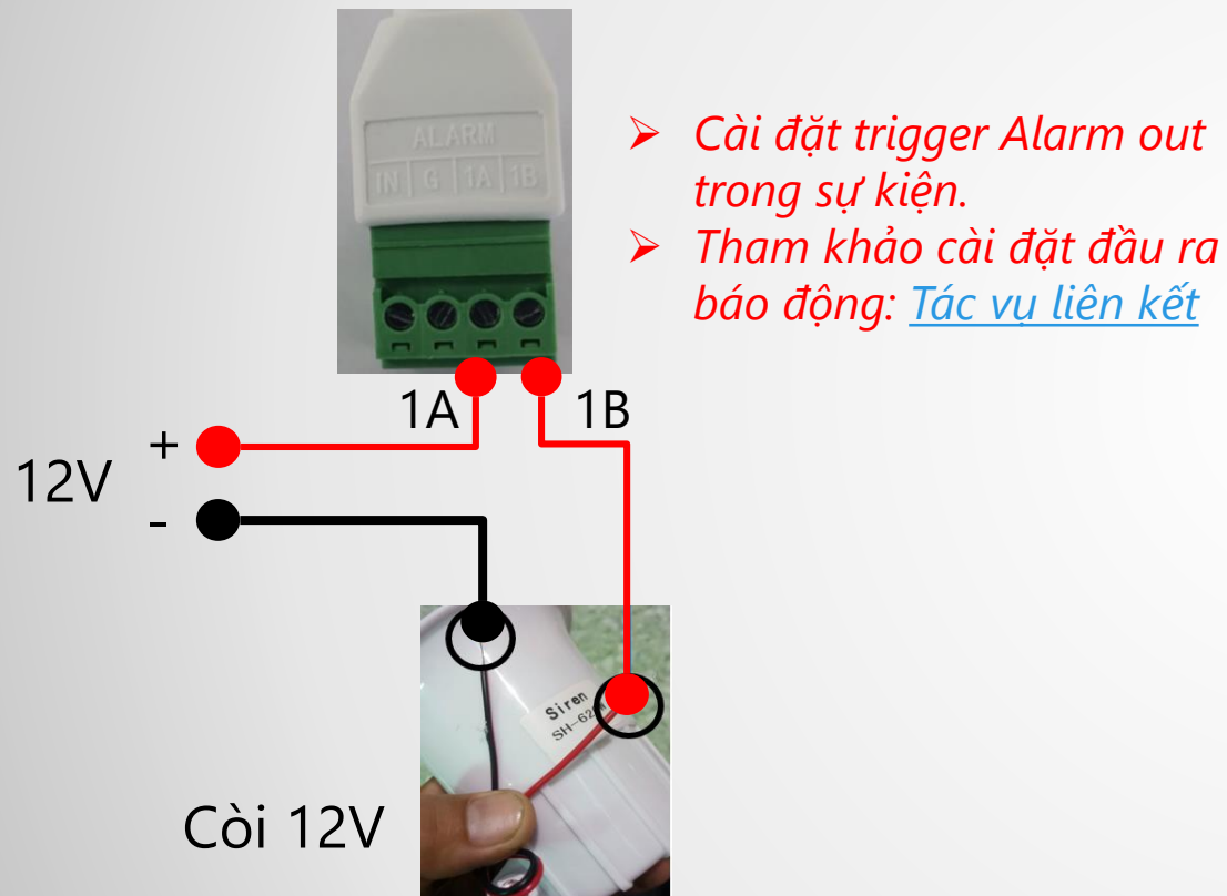
Đấu dây còi hú 12V
